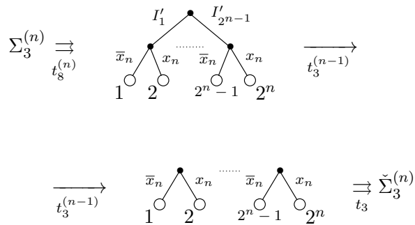
Рис. 7.10: вывод t_3^{(n)}
