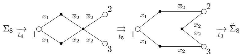
Рис. 7.4: вывод t_8
