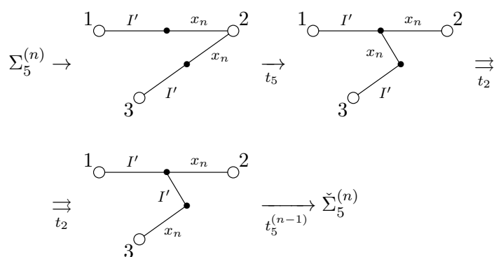
Рис. 7.12: вывод t_5^{(n)}
