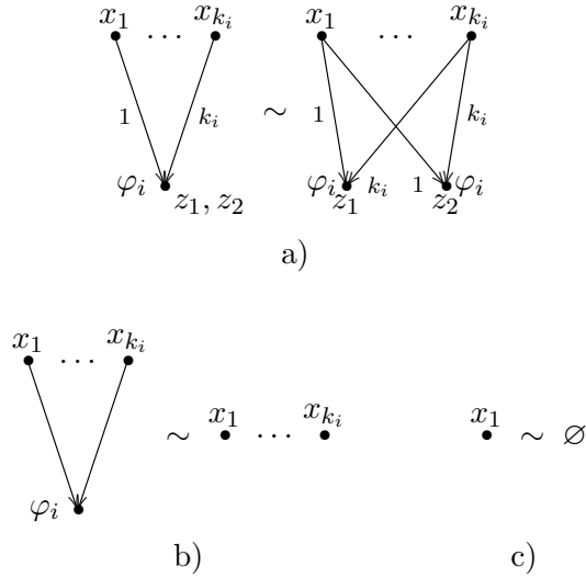
Рис. 5.2: тождества ветвления, снятия \Phi\Theta и снятия входа
