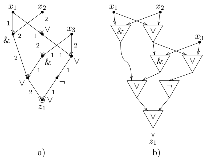
Рис. 4.2: СФЭ, полученная из квазидерева на рис. 3.2b
