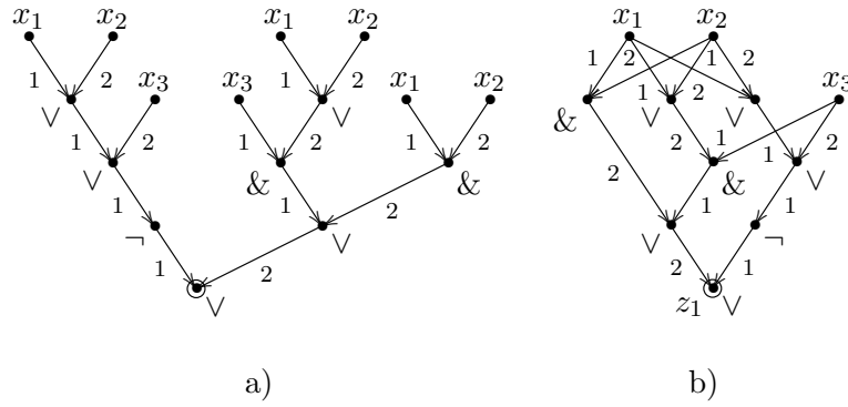
Рис. 3.2: представление формулы (3.1) деревом и квазидеревом
