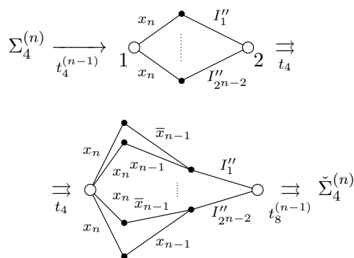
Рис. 7.11: вывод t_4^{(n)}
