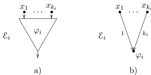
Рис. 4.1: функциональный элемент \mathcal{E}_i
