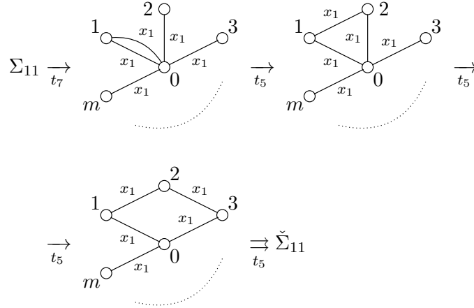
Рис. 7.7: вывод t_{11}
