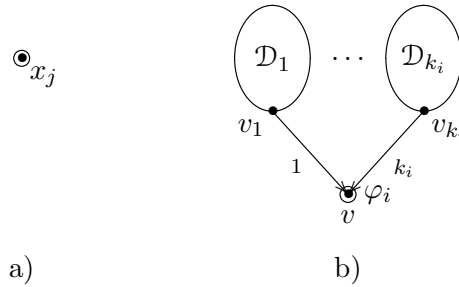
Рис. 3.1: представление формулы деревом
