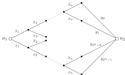
Рис. 2.1: \pi -схема для мультиплексорной функции
