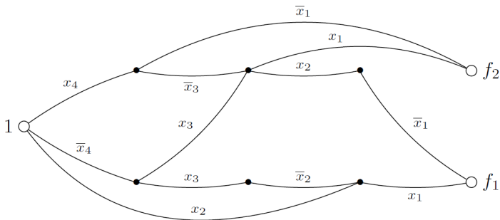
Рис. 3.4: пример КС, построенной методом каскадов
