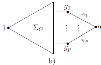
Рис. 7.1: Корректная реализация дизъюнкции ФАЛ g_1, \dots, g_p в классах КВС и ИКС
