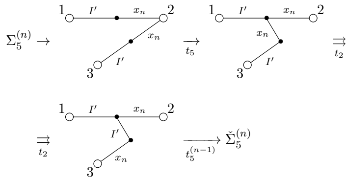
Рис. 7.12: вывод t_5^{(n)}
