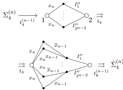
Рис. 7.11: вывод t_4^{(n)}
