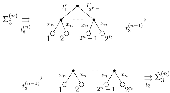
Рис. 7.10: вывод t_3^{(n)}
