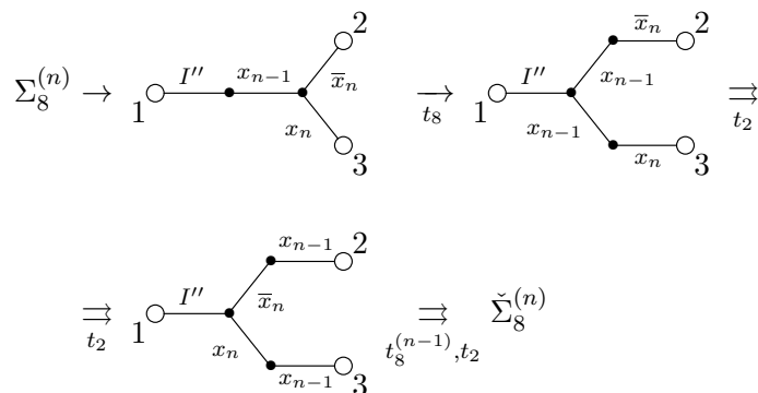
Рис. 7.9: вывод t_8^{(n)}
